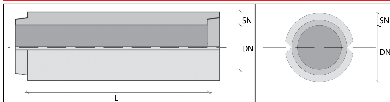
SEZ. LONGITUDINALE
